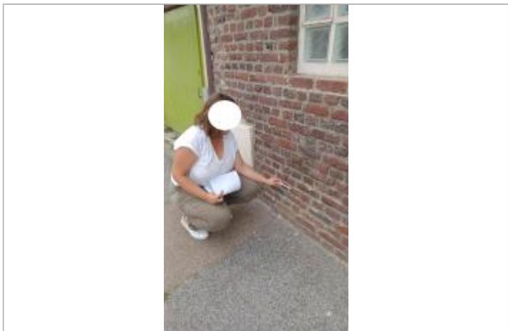
Laisse de crue au niveau de la 5ème rangée de briques.
