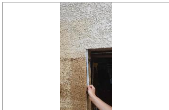
Laisse de crue sur mur jouxtant le garage à 9 cm du haut de l'ouverture du garage.
