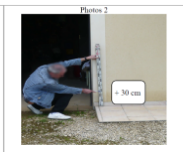
Trace du maximum de la crue sur la façade de la maison du 8 ter Rue Jules Vernes
