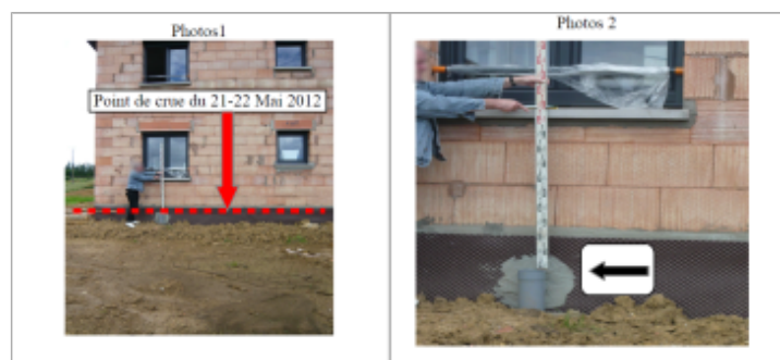
Trace du maximum de la crue sur le sous bassement de la maison en construction
