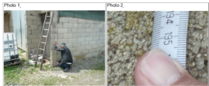
Trace du maximum de la crue sur la mur aggro du hangar
