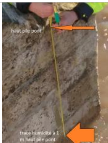
trace_humidité_1m_du_haut_pile_pont_seulle_CREULLY_DDTM14
