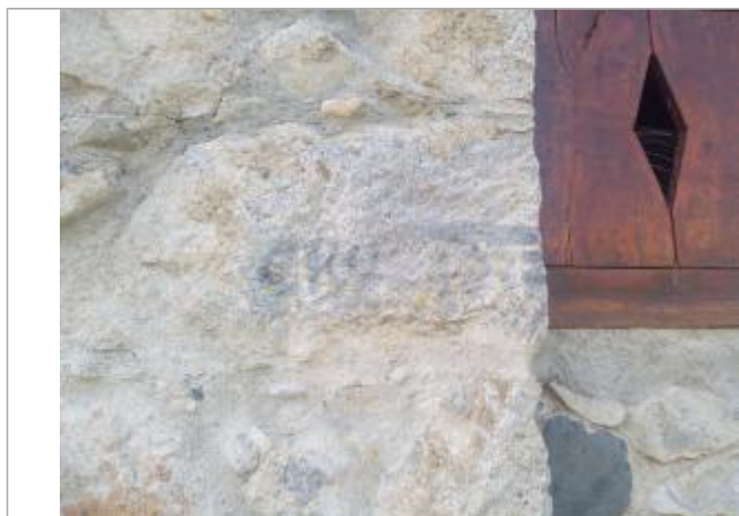
Trait de peinture reportant la PHE de la crue du 19 mai 1977
