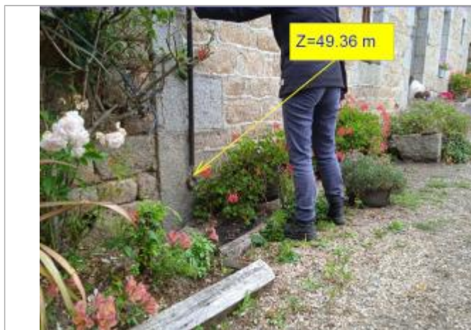
Repère lors du nivellement de 2022
